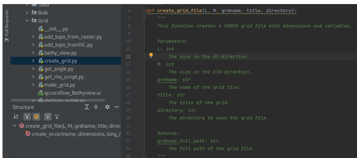
FIGURE 22 – Extrait du script du fichier create_grid.py pour la création initiale du fichier au format NetCDF.
